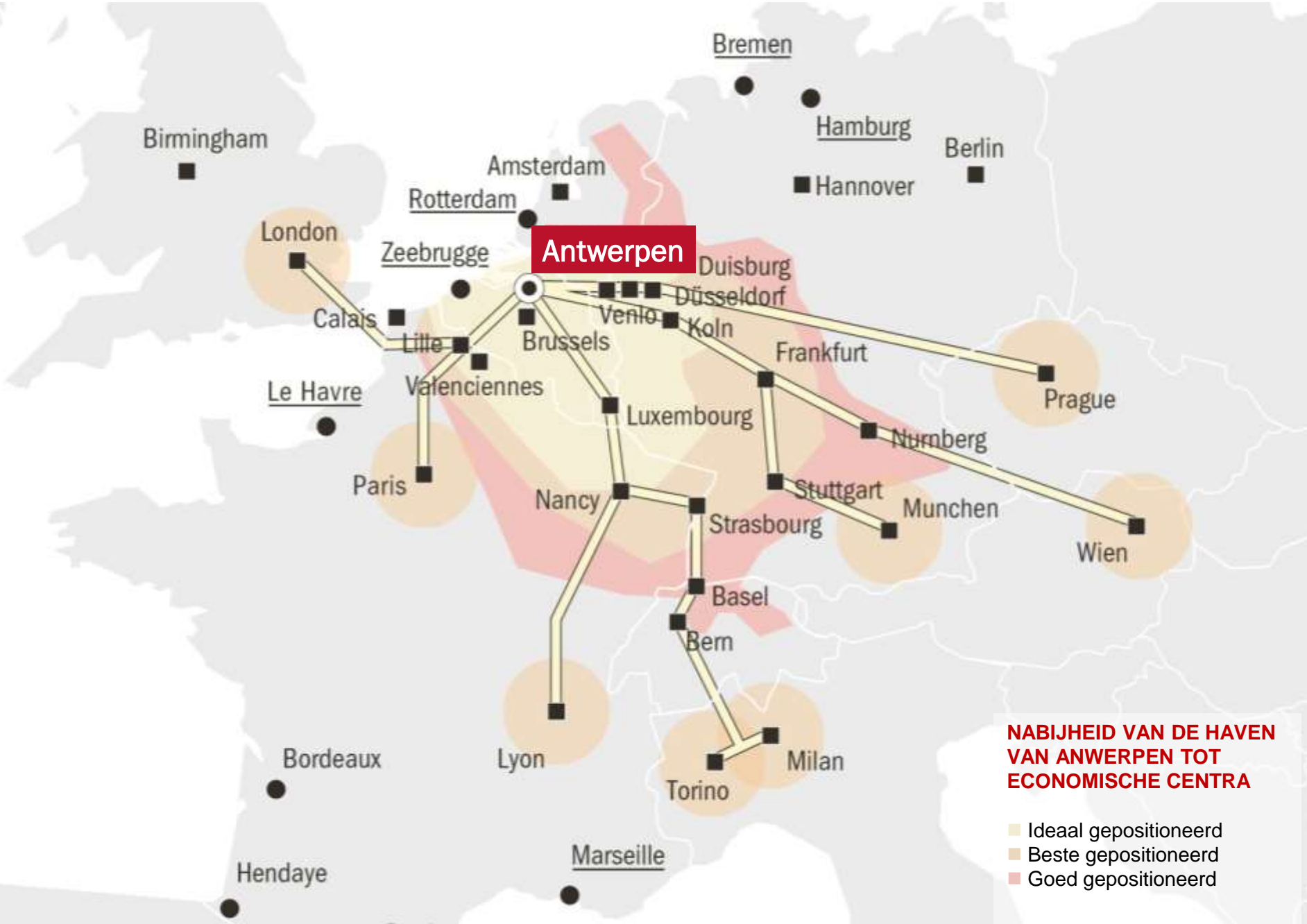
Het natuurlijke hinterland van de haven van Antwerpen
